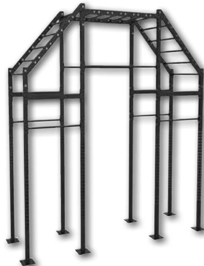
55079000 Estructura Funcional BR-4R464 Alto: 3,65 m. Ancho: 4,05. Largo: 1,20 m.
